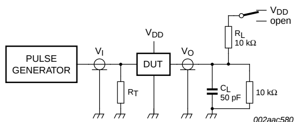
Fig 17. Test circuitry for enable/disable times, SDOUT ( t_{en}(SDOUT) and t_{dis}(SDOUT) )
